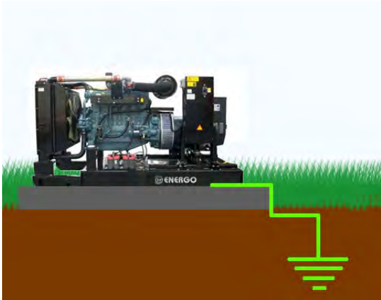
Типовое задание №2. Произвести защитное заземление ДВС
